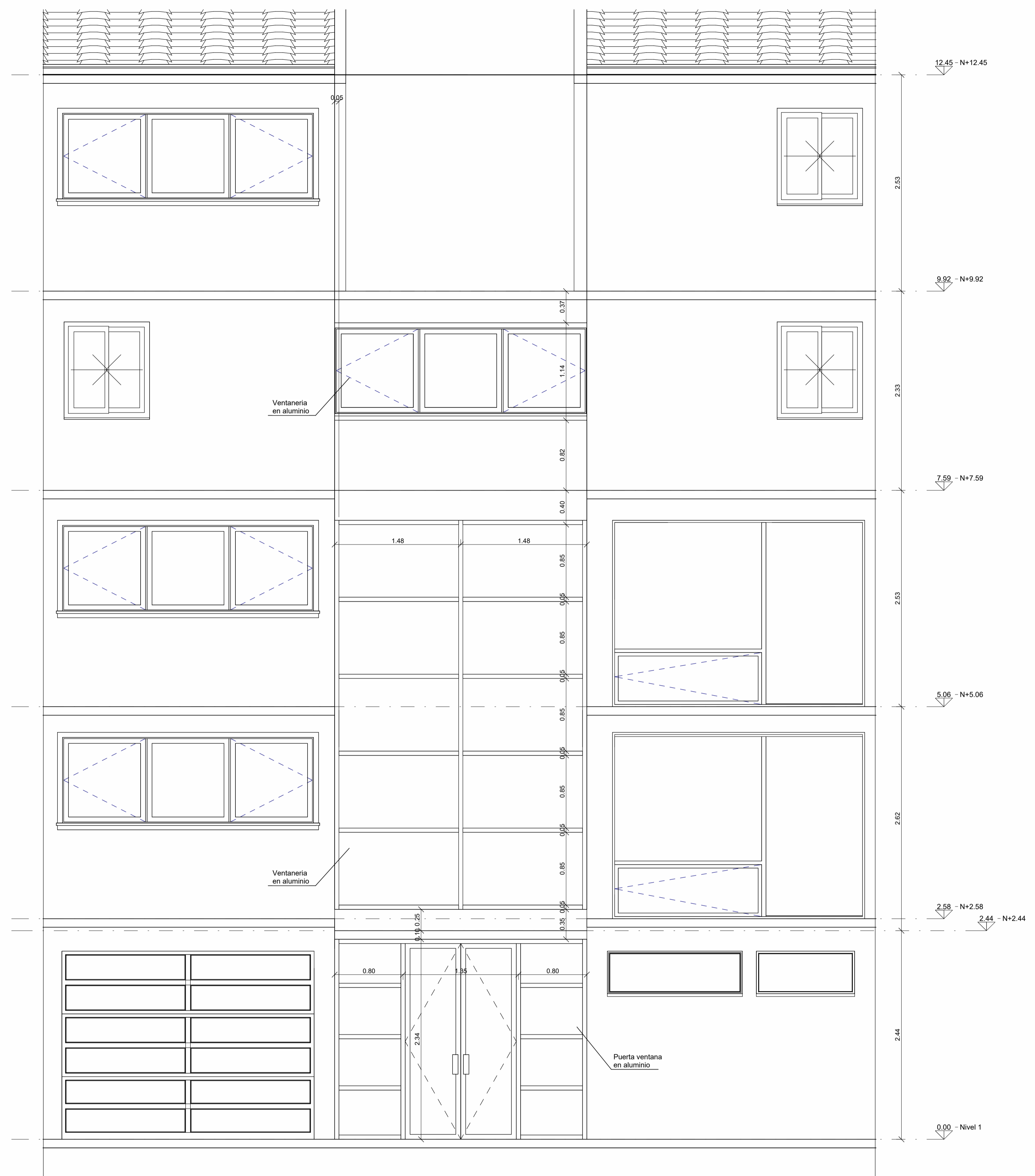
VISTA FRONTAL ESCALA 1:50
