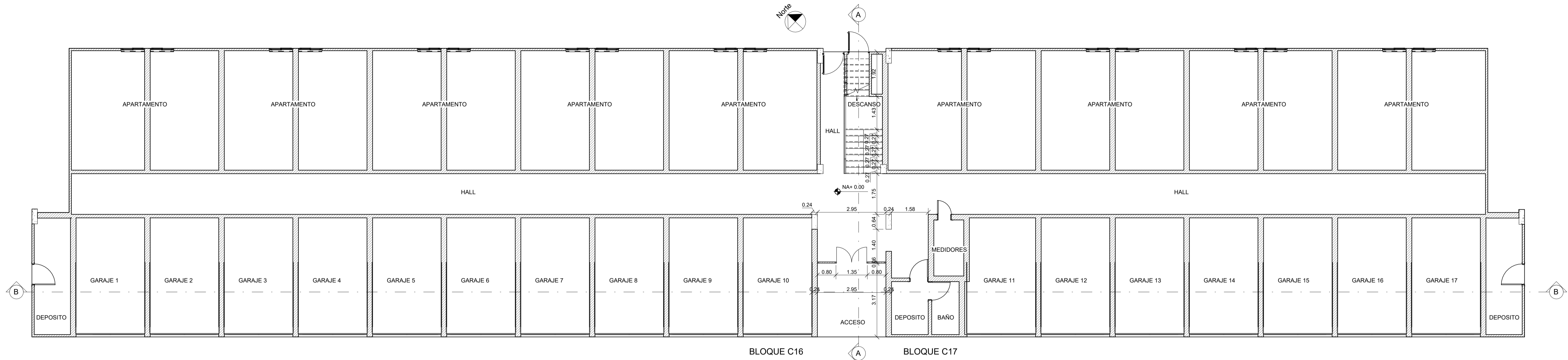
PLANTA DE PRIMER PISO ESCALA 1:75
